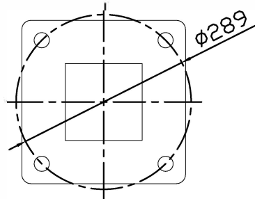
TEMPLATE (3:1)
